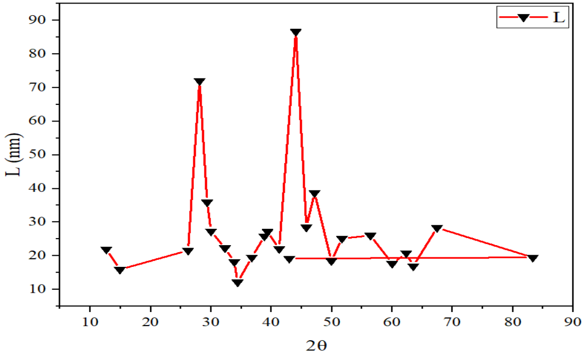
الشكل 7. يوضح الحجم البلوري مع (2 \theta ) للسمنت المقاوم
