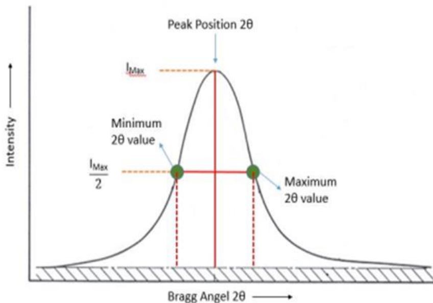
الشكل 6. قيمة الحد الأدنى (2\theta) والحد الأقصى لقيمة (2\theta) و نصف الحد الأقصى للقيم (FWHM) (Fatimah et al., 2022).
