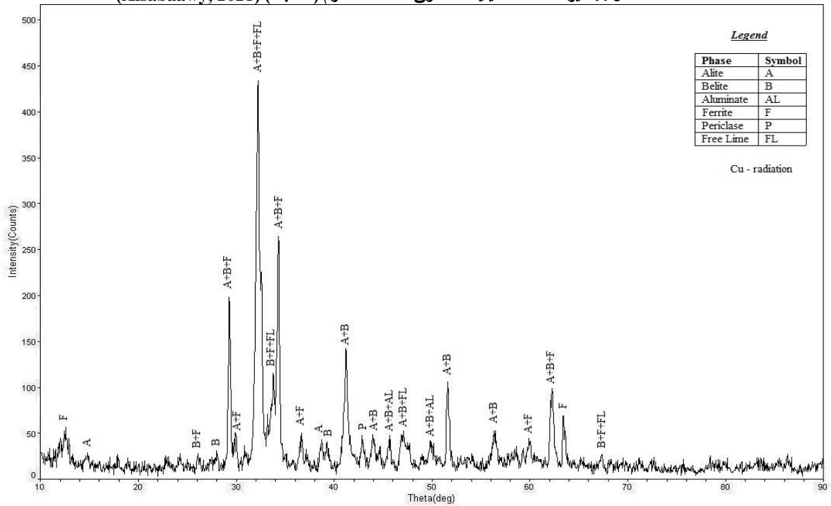
الشكل 4. حيود الأشعة السينية لمسحوق أسمنت المقاوم (الحدباء) (Alsabaawy, 2021)
