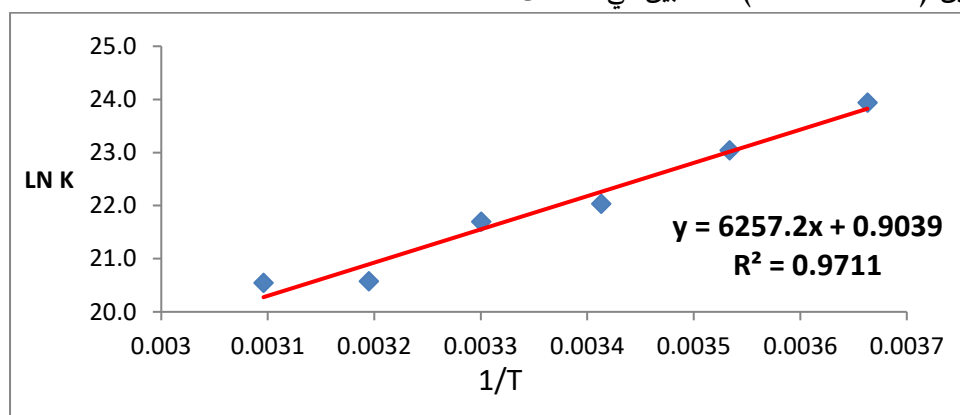
الشكل (١) العلاقة البيانية بين ( \ln K ) ضد ( 1/T ) للصبغة APNPP + o-phDA عند الدالة الحامضية الطبيعية.
