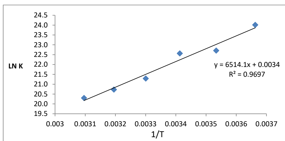
الشكل (٤) العلاقة البيانية بين (LnK) ضد (T\1) للصبغة DCPPP + o-phDA عند الدالة الحامضية الطبيعية.
