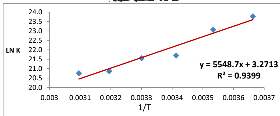
الشكل (٢) العلاقة البيانية بين ( \ln K ) ضد ( 1/T ) للصبغة APHPP + o-phDA
