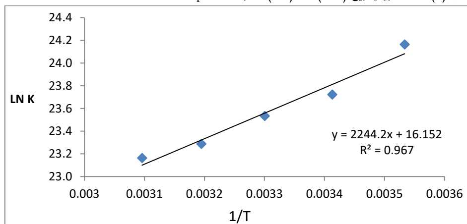
الشكل (٥) العلاقة البيانية بين (LnK) ضد (T\1) للصبغة APNPe + o-phDA عند الدالة الحامضية الطبيعية.
