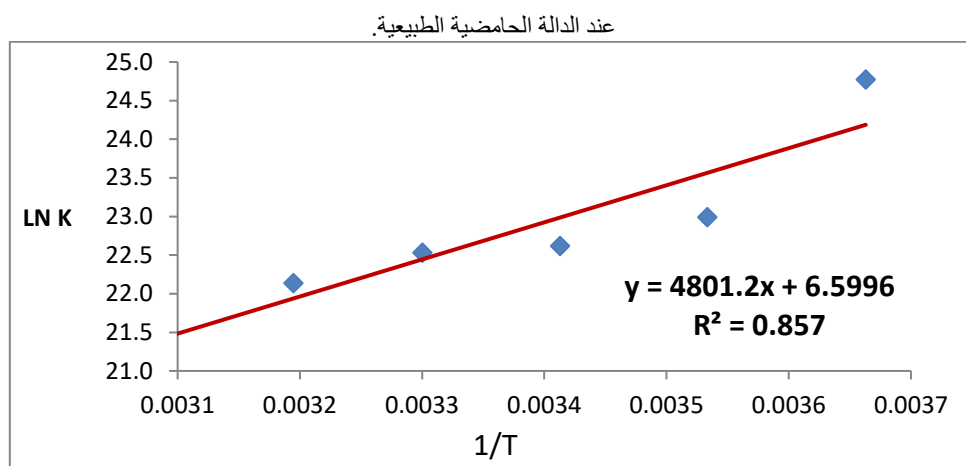
الشكل (٣) العلاقة البيانية بين (LnK) ضد (T\1) للصبغة CPPP + o-phDA عند الدالة الحامضية الطبيعية.
